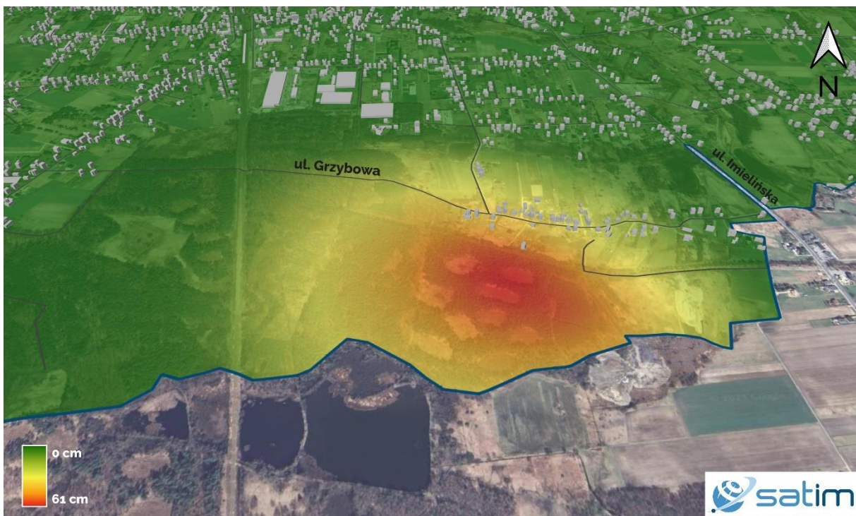
Ryc. 7 - Wizualizacja budynków na niecce obniżeniowej. Kolorami oznaczone zostały budynki ze względu na wielkość osiadania terenu pod nimi w I półroczu 2024 r.
