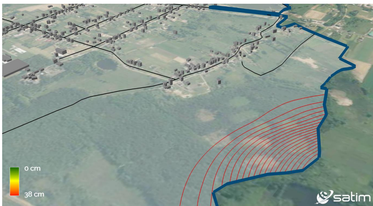
Ryc. 8 – Wizualizacja budynków na niecce obniżeniowej. Kolorami oznaczone zostały budynki ze względu na wielkość osiadania terenu pod nimi w I kwartale 2022 r. Izolinie osiadań oddalone od siebie o stałą wartość 2 cm cięcia poziomowego
