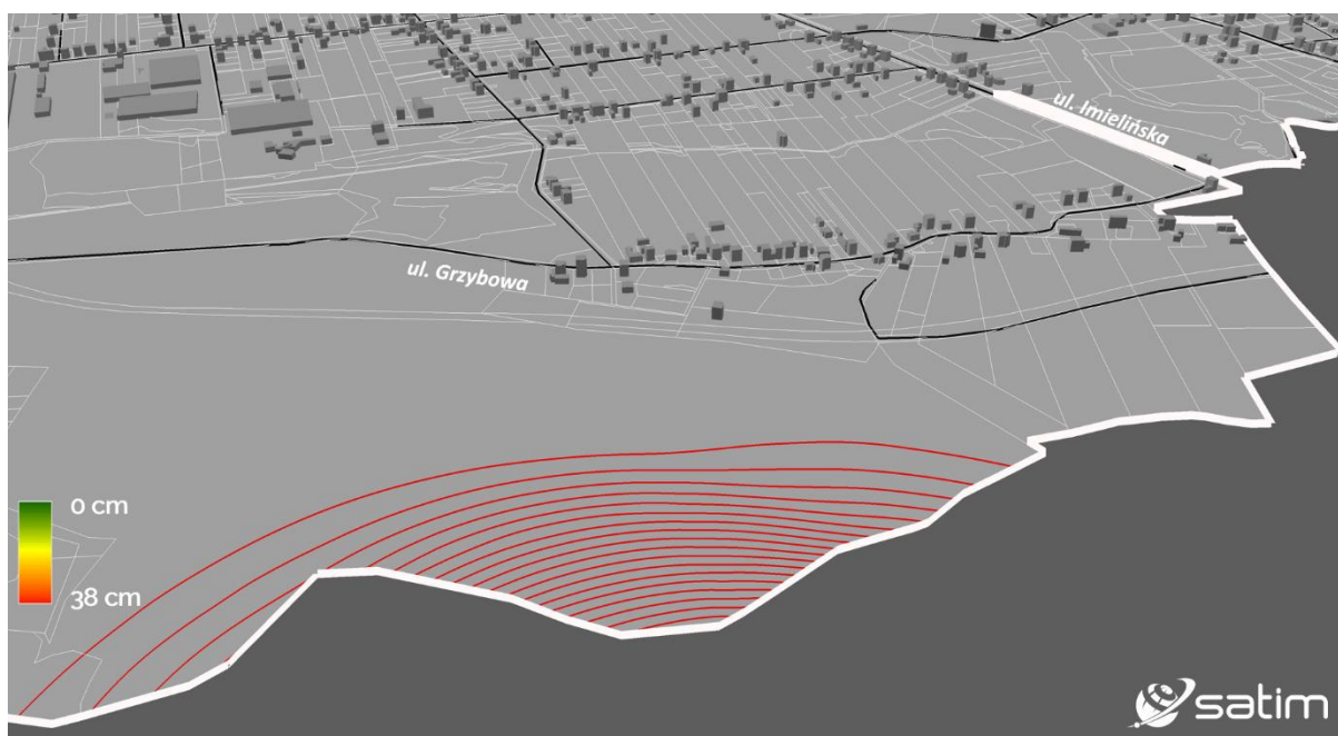
Ryc. 10 – Wizualizacja budynków i ulic. Kolorami oznaczone zostały budynki ze względu na wielkość osiadania terenu pod nimi w I kwartale 2022 r. Izolinie osiadań oddalone od siebie o stałą wartość 2 cm cięcia poziomicowego
