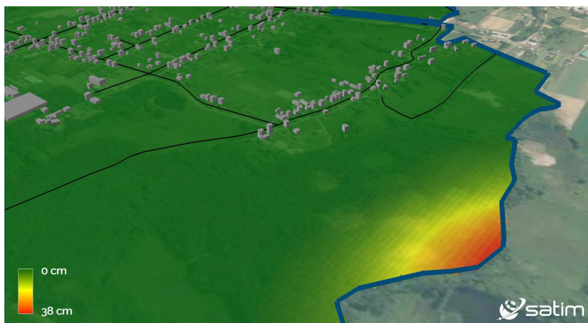
Ryc. 7 - Wizualizacja budynków na niecce obniżeniowej. Kolorami oznaczone zostały budynki ze względu na wielkość osiadania terenu pod nimi w I kwartale 2022 r.
