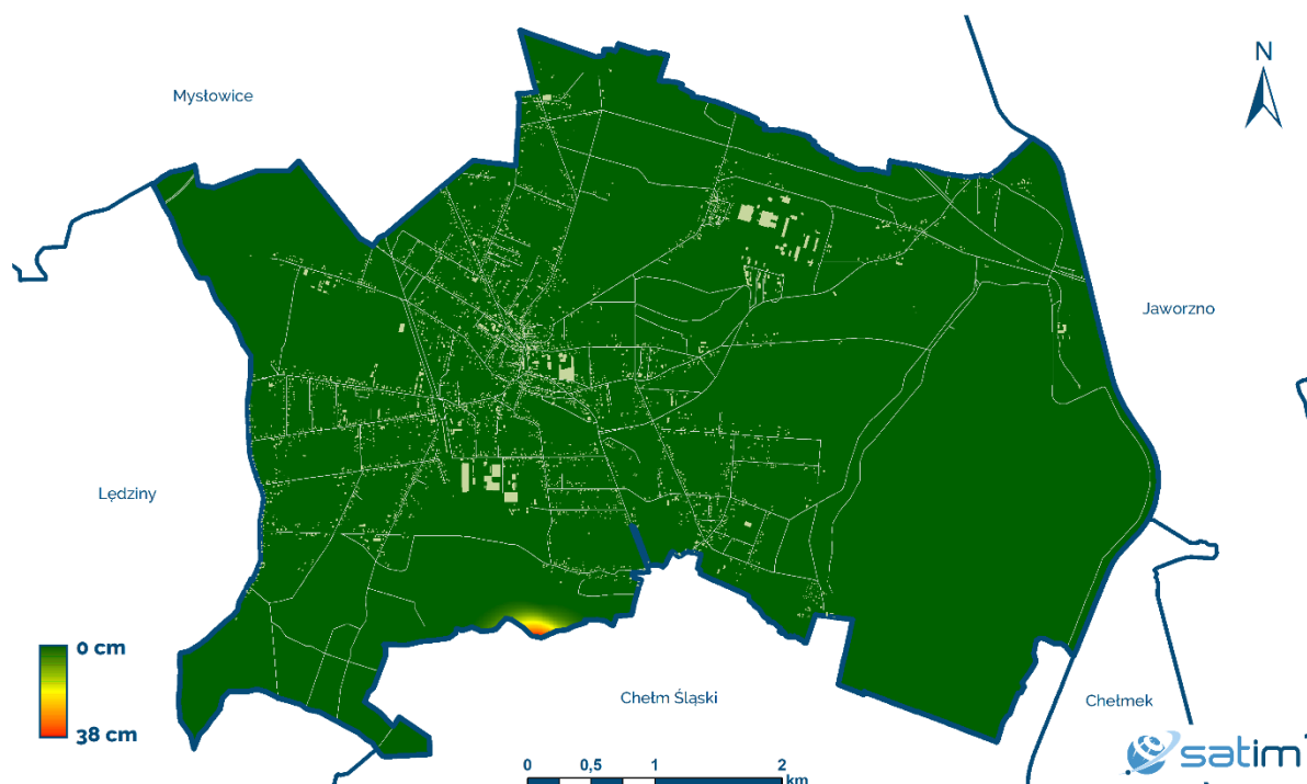
Ryc. 1 – Mapa pionowych przemieszczeń terenu. Maksymalne osiadania terenu, jakie wystąpiły w I kwartale 2022 roku to ok. 38 cm.
