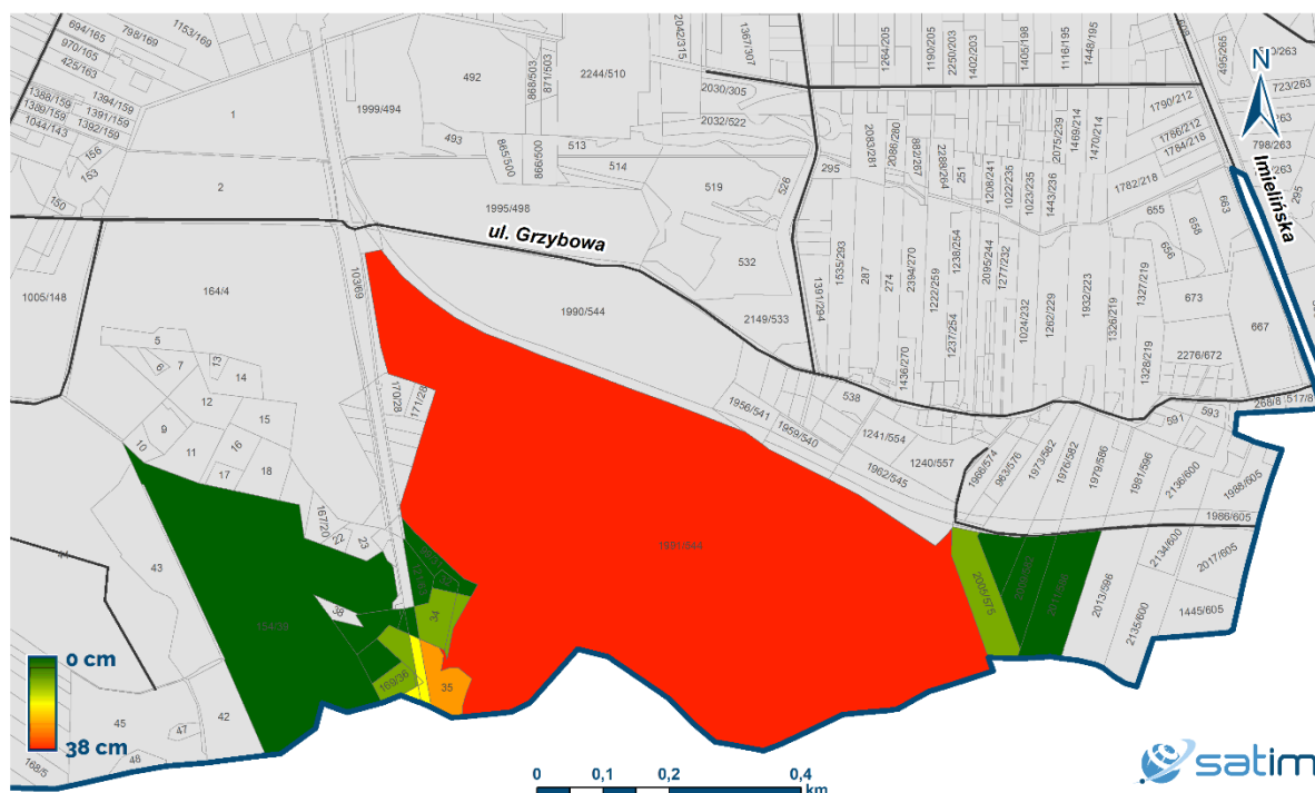
Ryc. 6 - Mapa działek ewidencyjnych. Kolorami oznaczone zostały działki ze względu na maksymalną wielkość osiadania terenu w ich obrębie.
