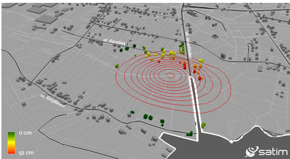
Ryc. 10 – Wizualizacja budynków i ulic. Kolorami oznaczone zostały budynki ze względu na wielkość osiadania terenu pod nimi w I kwartale 2021 r. Izolinie osiadań oddalone od siebie o stałą wartość 5 cm cięcia poziomowego
