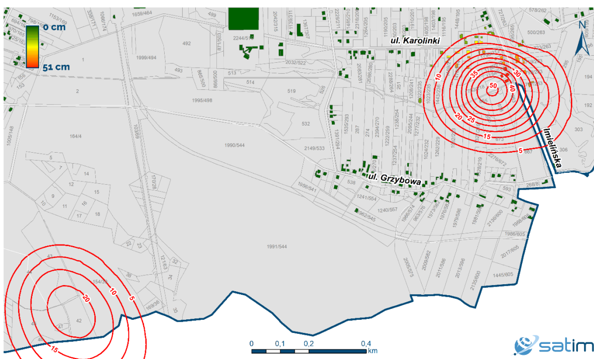
Ryc. 4 - Mapa pionowych przemieszczeń terenu – obniżenia w formie izolinii. Izolinie oddalone od siebie o stałą wartość 5 cm cięcia poziomowego. W I kwartale 2021 r. 44 budynki znajdowały się na zagrożonym obszarze.
