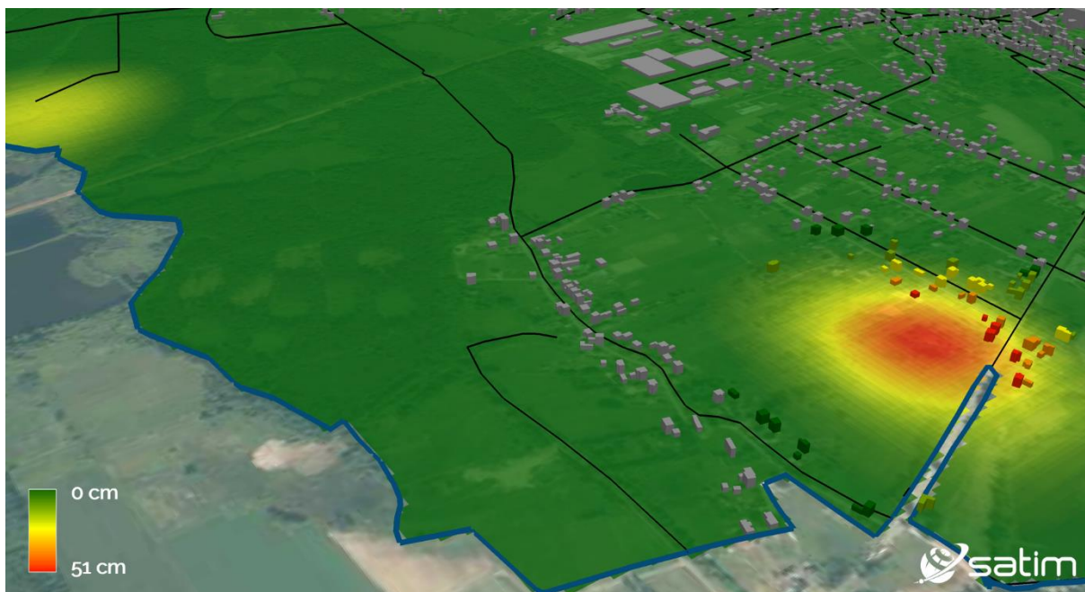
Ryc. 7 – Wizualizacja budynków na niecce obniżeniowej. Kolorami oznaczone zostały budynki ze względu na wielkość osiadania terenu pod nimi w I kwartale 2021 r.
