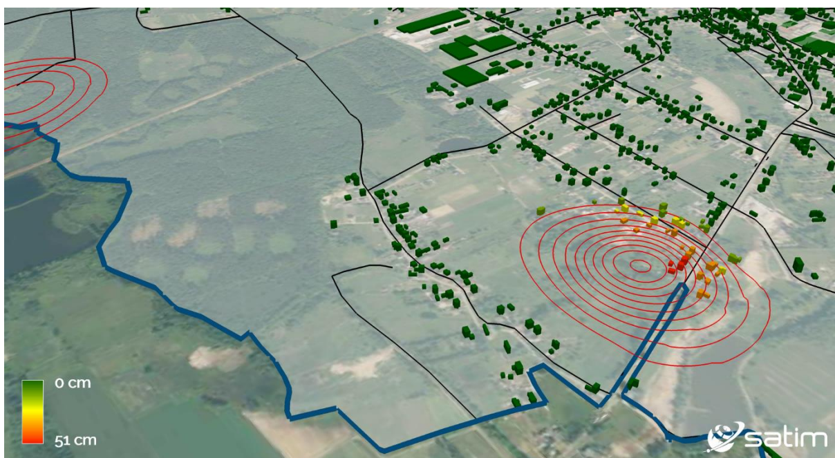
Ryc. 8 – Wizualizacja budynków na niecce obniżeniowej. Kolorami oznaczone zostały budynki ze względu na wielkość osiadania terenu pod nimi w I kwartale 2021 r. Izolinie osiadań oddalone od siebie o stałą wartość 5 cm cięcia poziomowego
