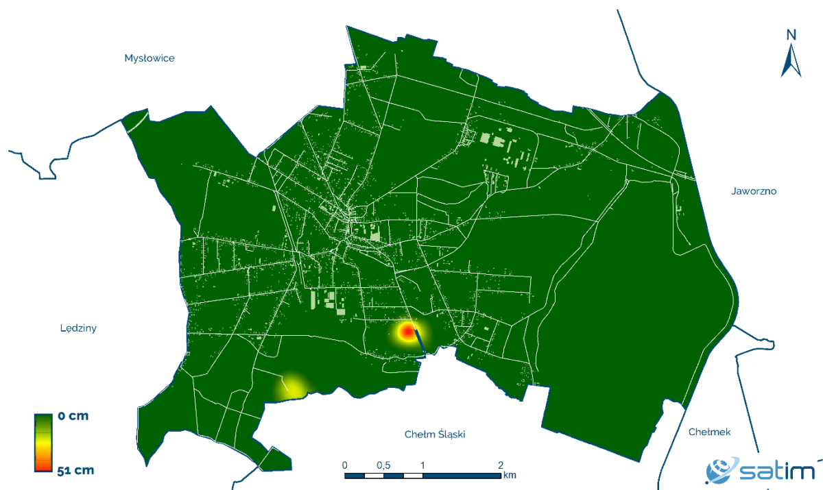
Ryc. 1 – Mapa pionowych przemieszczeń terenu. Maksymalne osiadania terenu jakie wystąpiły w I kwartale 2021 roku to ok. 51 cm.
