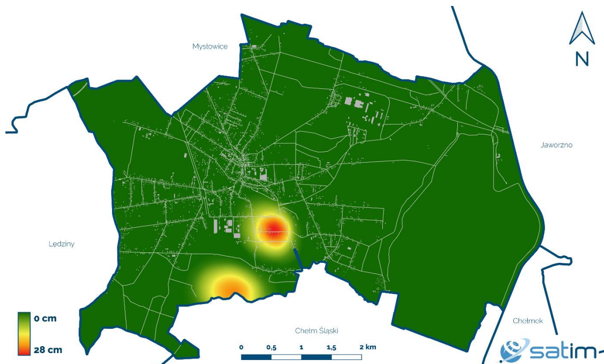
Ryc. 1 – Mapa pionowych przemieszczeń terenu. Maksymalne osiadania terenu, jakie wystąpiły w IV kwartale 2022 roku to ok. 28 cm.
