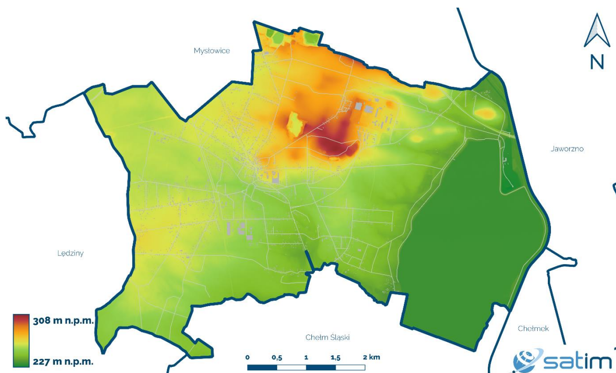
Ryc. 7 – Numeryczny model terenu po aktualizacji (stan na 10.12.2022); od NMT z 2022 roku odjęte zostały wartości osiadań jakie wystąpiły w okresie od stycznia 2022 do grudnia 2022 r.
