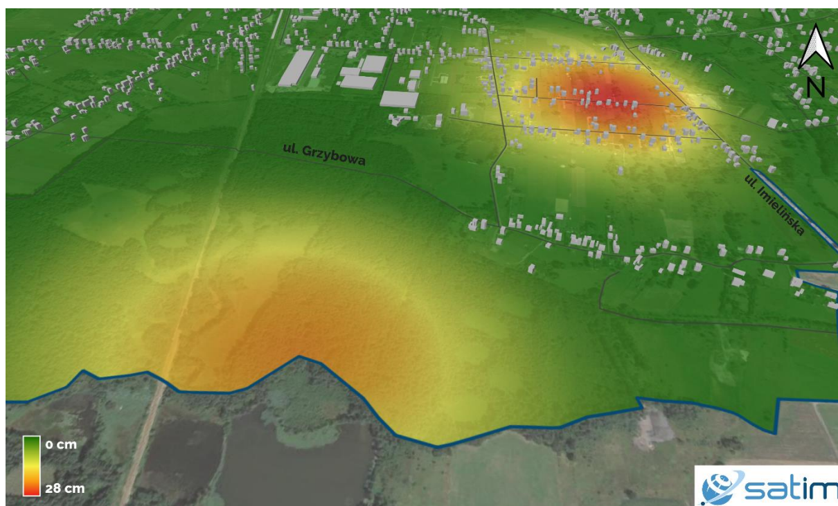
Ryc. 8 – Wizualizacja budynków na niecce obniżeniowej. Kolorami oznaczone zostały budynki ze względu na wielkość osiadania terenu pod nimi w IV kwartale 2022 r.
