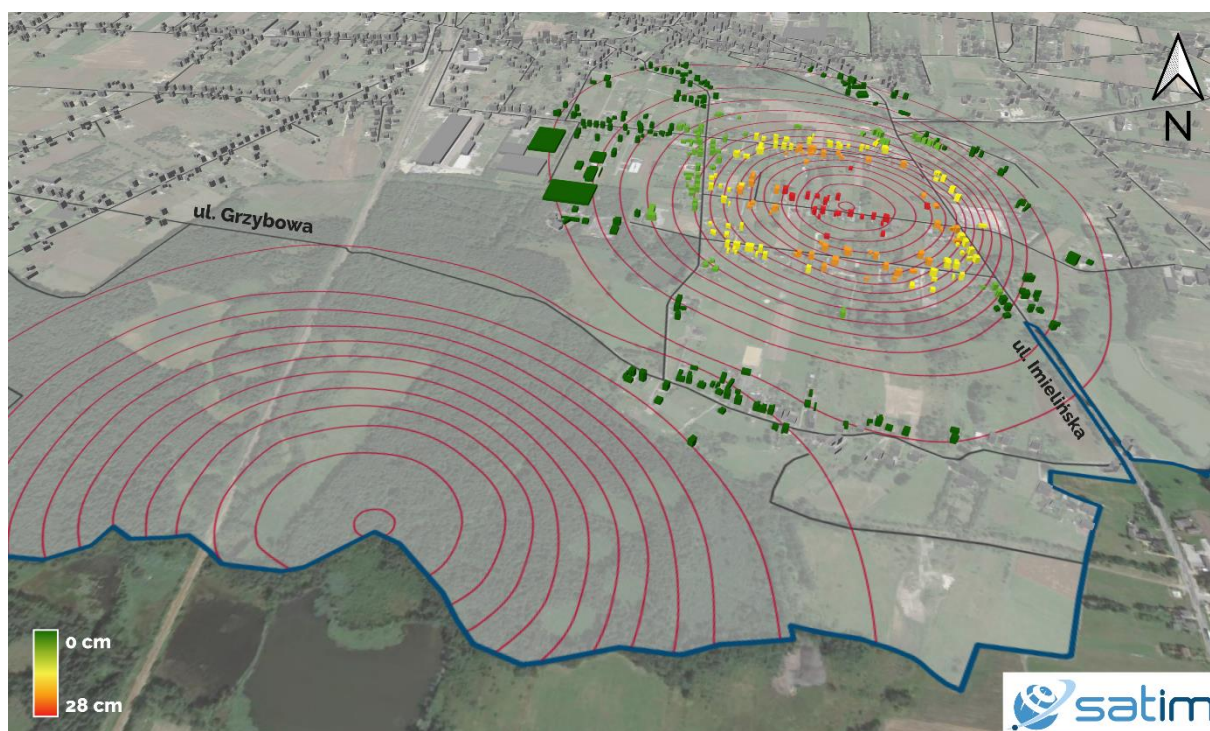
Ryc. 9 – Wizualizacja budynków na niecce obniżeniowej. Kolorami oznaczone zostały budynki ze względu na wielkość osiadania terenu pod nimi w IV kwartale 2022 r. Izolinie osiadań oddalone od siebie o stałą wartość 2 cm cięcia poziomowego.
