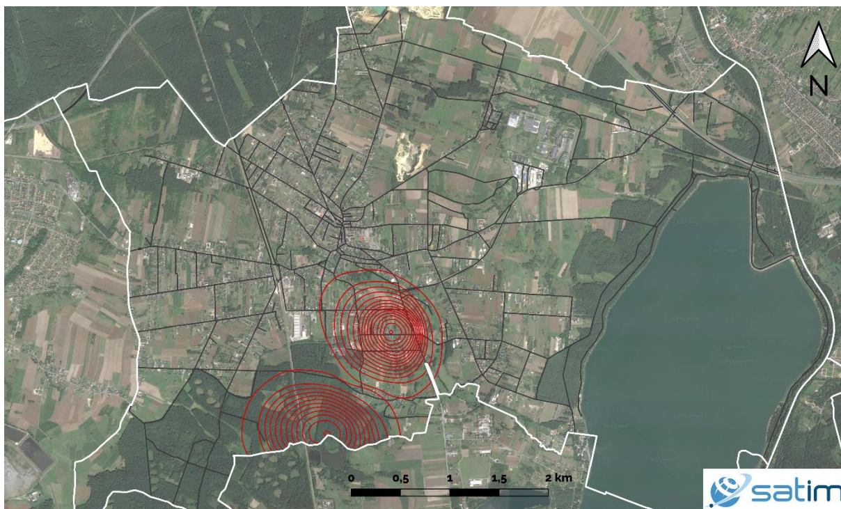
Ryc. 12 – Wizualizacja osiadań terenu gminy Imielin z ortofotomapą w podkładzie.
