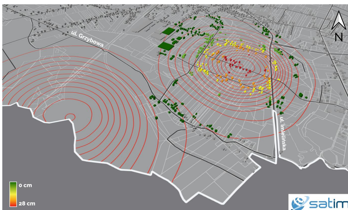
Ryc. 11 – Wizualizacja budynków i ulic. Kolorami oznaczone zostały budynki ze względu na wielkość osiadania terenu pod nimi w IV kwartale 2022 r. Izolinie osiadań oddalone od siebie o stałą wartość 2 cm cięcia poziomicowego.
