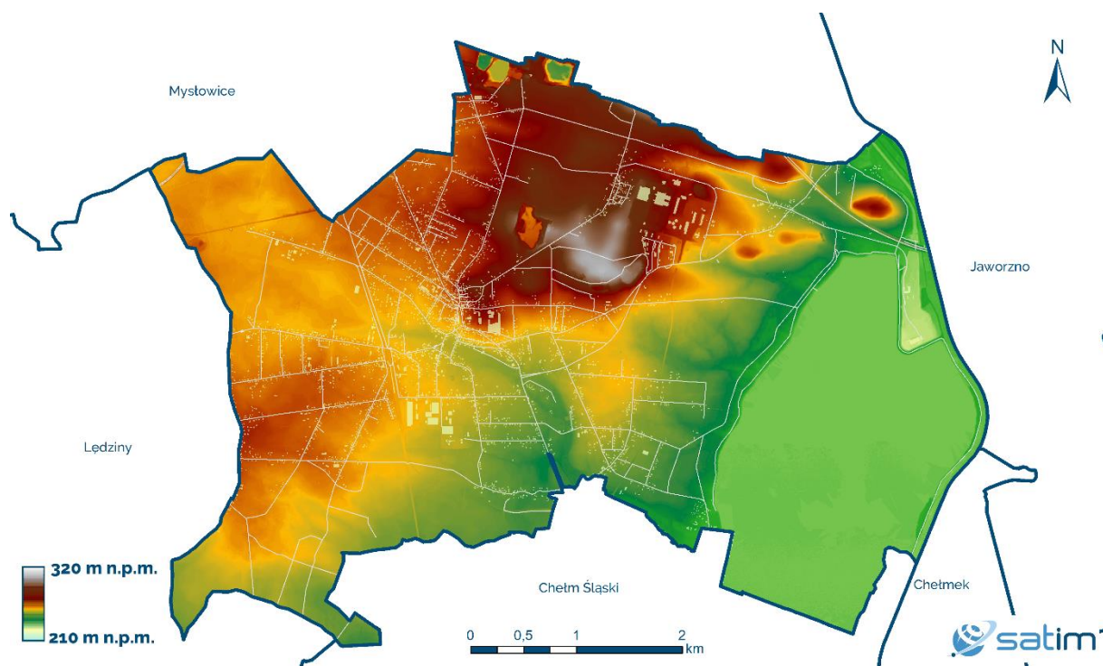
Ryc. 7 – Numeryczny model terenu po aktualizacji (stan na 01.01.2021); od NMT z 2020 roku odjęte zostały wartości osiadań jakie wystąpiły w okresie od stycznia 2019 do końca grudnia 2020 r.
