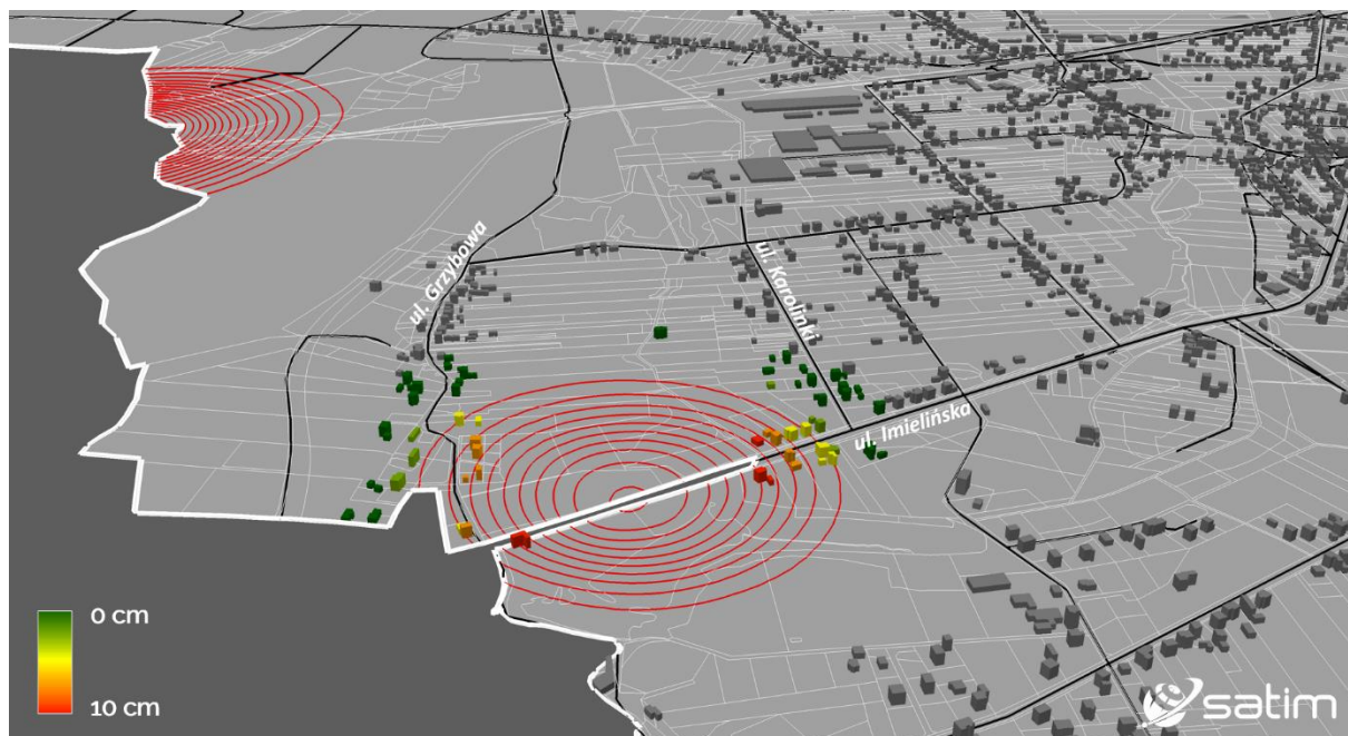
Ryc. 11 – Wizualizacja budynków i ulic. Kolorami oznaczone zostały budynki ze względu na wielkość osiadania terenu pod nimi w IV kwartale 2020 r. Izolinie osiadań oddalone od siebie o stałą wartość 2 cm cięcia poziomicowego
