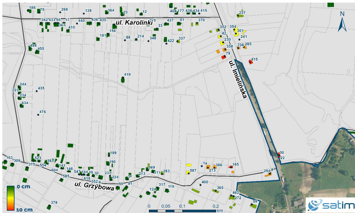
Ryc. 5 - Mapa zagrożonych budynków. Kolorami oznaczone zostały budynki ze względu na wielkość osiadania terenu pod nimi w IV kwartale 2020 r.; liczby przy budynkach oznaczają numery adresowe
