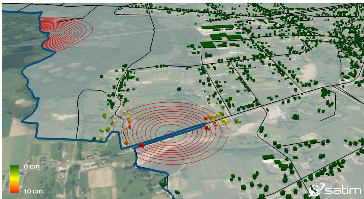
Ryc. 9 – Wizualizacja budynków na niecce obniżeniowej. Kolorami oznaczone zostały budynki ze względu na wielkość osiadania terenu pod nimi w IV kwartale 2020 r. Izolinie osiadań oddalone od siebie o stałą wartość 2 cm cięcia poziomowego
