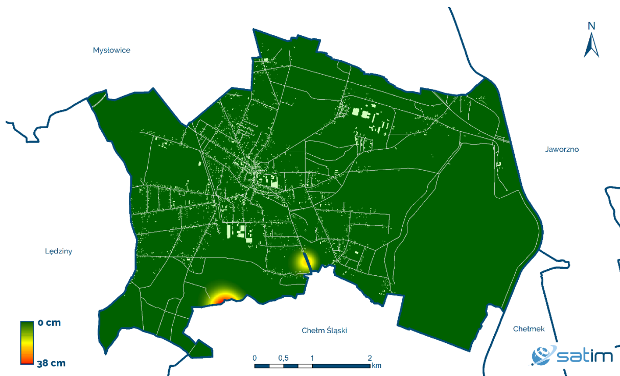
Ryc. 1 – Mapa pionowych przemieszczeń terenu. Maksymalne osiadania terenu, jakie wystąpiły w IV kwartale 2020 roku to ok. 38 cm.
