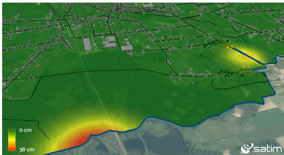
Ryc. 8 – Wizualizacja budynków na niecce obniżeniowej. Kolorami oznaczone zostały budynki ze względu na wielkość osiadania terenu pod nimi w IV kwartale 2020 r.
