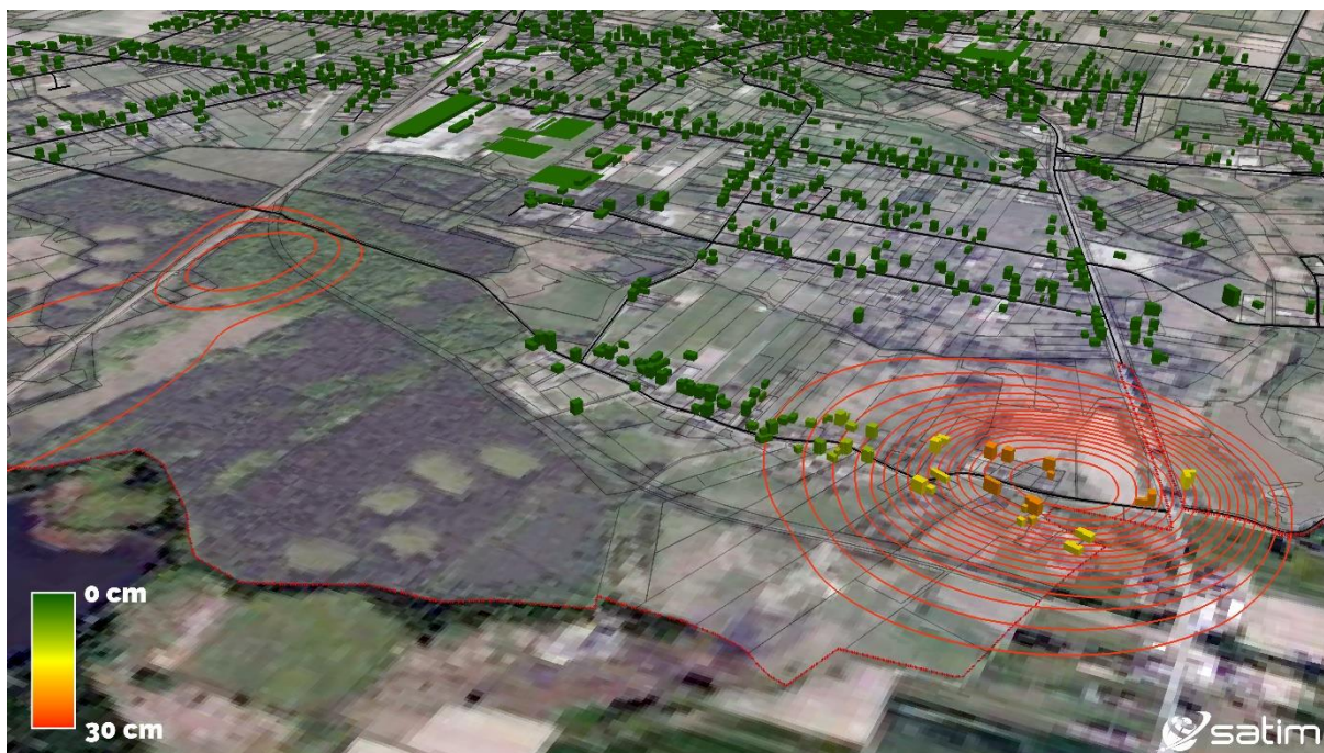
Ryc. 9 – Wizualizacja budynków na niecce obniżeniowej; kolorami oznaczone zostały budynki ze względu na wielkość osiadania terenu pod nimi w IV kwartale 2019 r. (izolinie osiadań oddalone od siebie o stałą wartość 1 cm cięcia poziomicowego)
