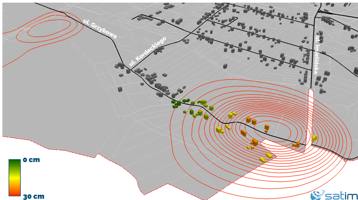
Ryc.11 – Wizualizacja budynków i ulic; kolorami oznaczone zostały budynki ze względu na wielkość osiadania terenu pod nimi w IV kwartale 2019r. (izolinie osiadań oddalone od siebie o stałą wartość 1 cm cięcia poziomicowego)
