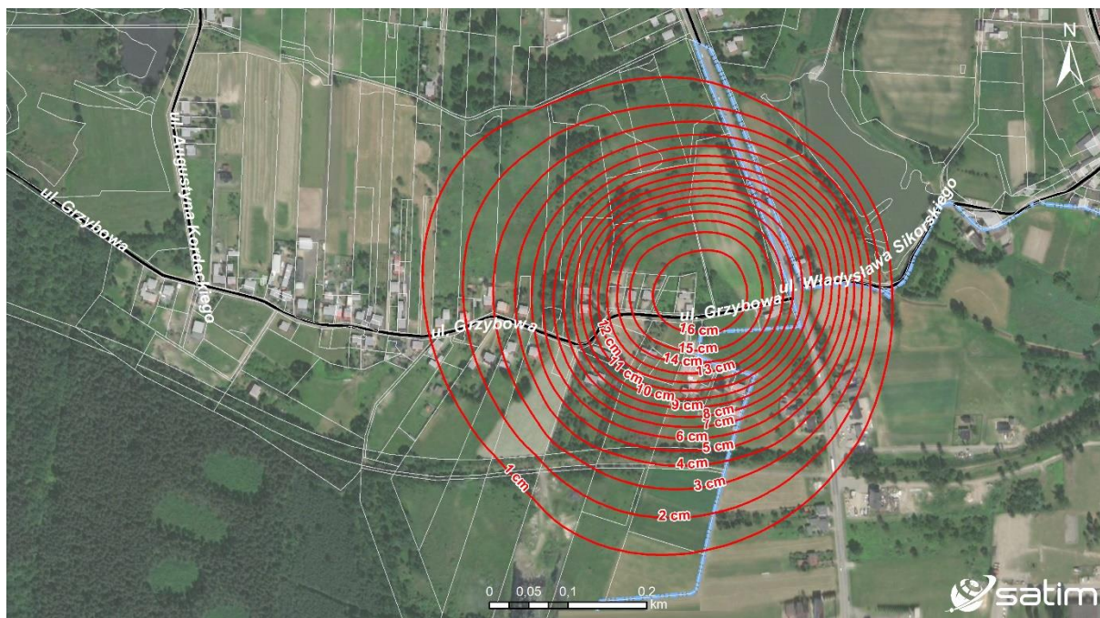
Ryc. 3 - Mapa pionowych przemieszczeń terenu – obniżenia w formie izolinii (izolinie oddalone od siebie o stałą wartość 1 cm cięcia poziomicowego)
