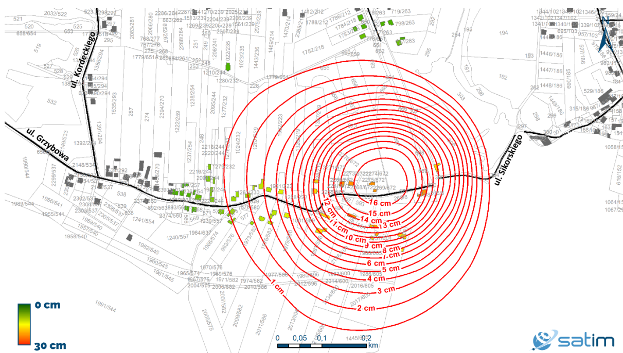
Ryc. 4 - Mapa pionowych przemieszczeń terenu – obniżenia w formie izolinii (izolinie oddalone od siebie o stałą wartość 1 cm cięcia poziomicowego)
