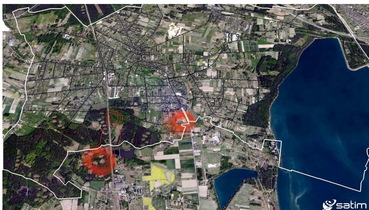
Ryc. 12 – Wizualizacja osiadań terenu gminy Imielin z ortofotomapą w podkładzie
