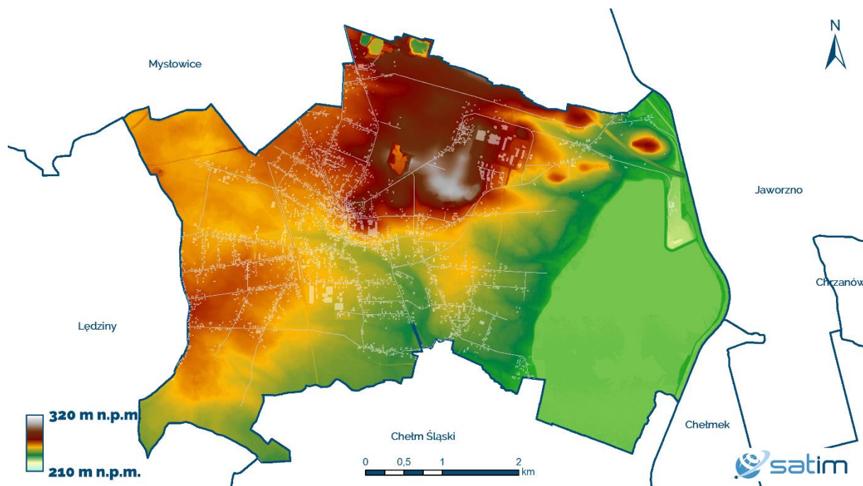
Ryc. 7 – Numeryczny model terenu po aktualizacji (stan na 01.01.2020); od NMT z 2019 roku odjęte zostały wartości osiadań jakie wystąpiły w okresie od stycznia 2019 do końca grudnia 2019 r.
