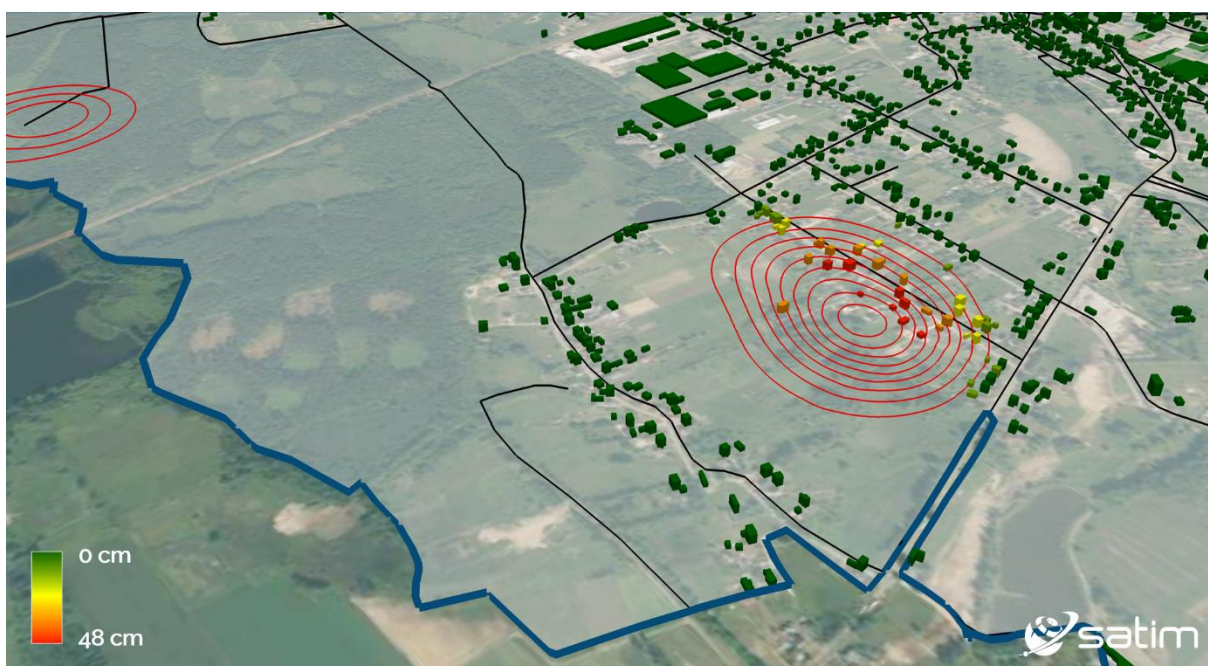
Ryc. 8 – Wizualizacja budynków na niecce obniżeniowej. Kolorami oznaczone zostały budynki ze względu na wielkość osiadania terenu pod nimi w II kwartale 2021 r. Izolinie osiadań oddalone od siebie o stałą wartość 5 cm cięcia poziomowego
