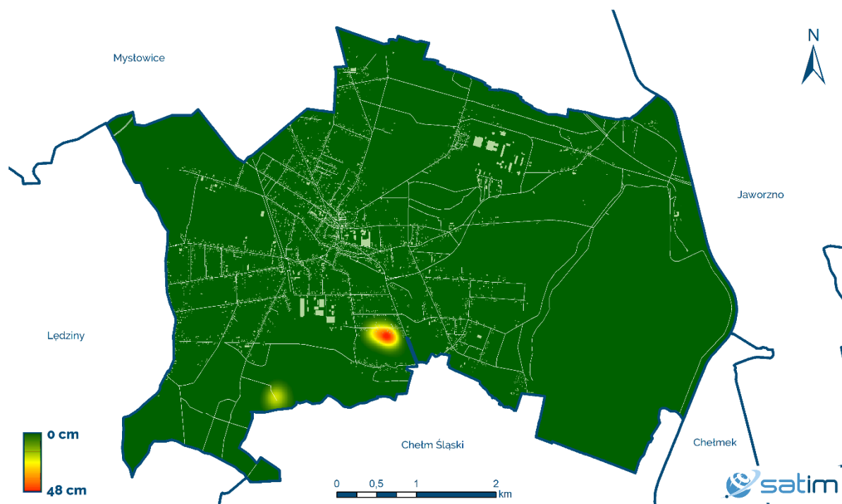
Ryc. 1 – Mapa pionowych przemieszczeń terenu. Maksymalne osiadania terenu jakie wystąpiły w II kwartale 2021 roku to ok. 48 cm.
