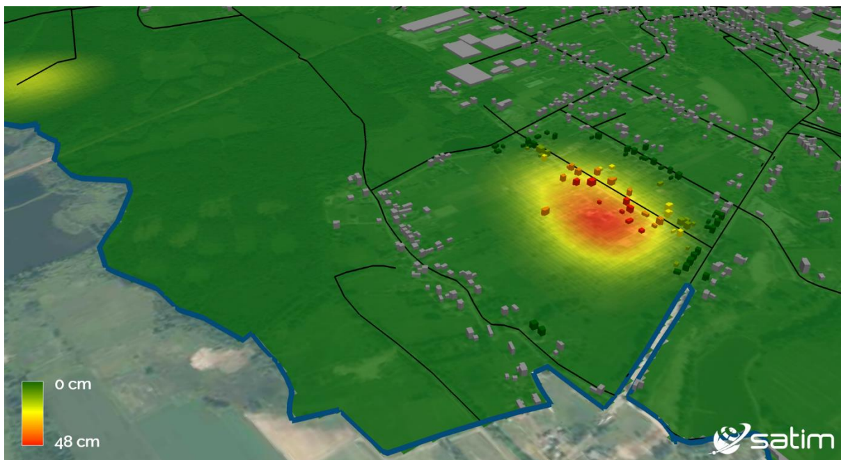
Ryc. 7 – Wizualizacja budynków na niecce obniżeniowej. Kolorami oznaczone zostały budynki ze względu na wielkość osiadania terenu pod nimi w II kwartale 2021 r.
