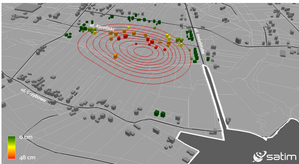
Ryc. 10 – Wizualizacja budynków i ulic. Kolorami oznaczone zostały budynki ze względu na wielkość osiadania terenu pod nimi w II kwartale 2021 r. Izolinie osiadań oddalone od siebie o stałą wartość 5 cm cięcia poziomowego
