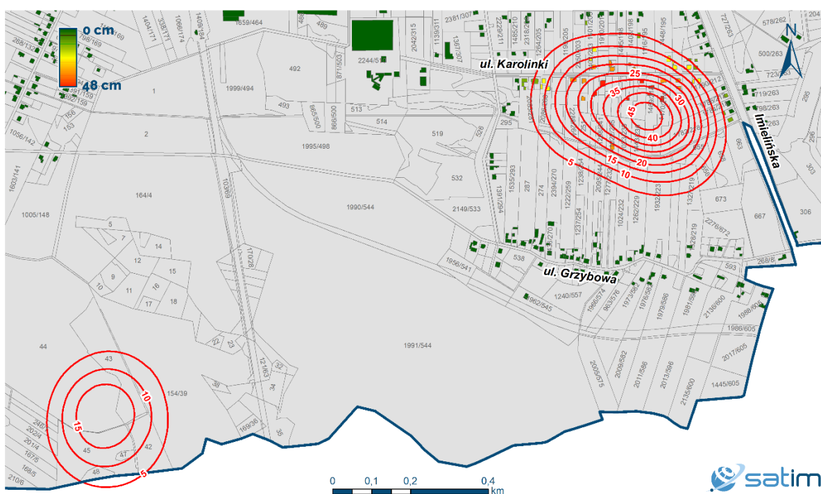
Ryc. 4 - Mapa pionowych przemieszczeń terenu – obniżenia w formie izolinii. Izolinie oddalone od siebie o stałą wartość 5 cm cięcia poziomowego. W II kwartale 2021 r. 62 budynki znajdowały się na zagrożonym obszarze.
