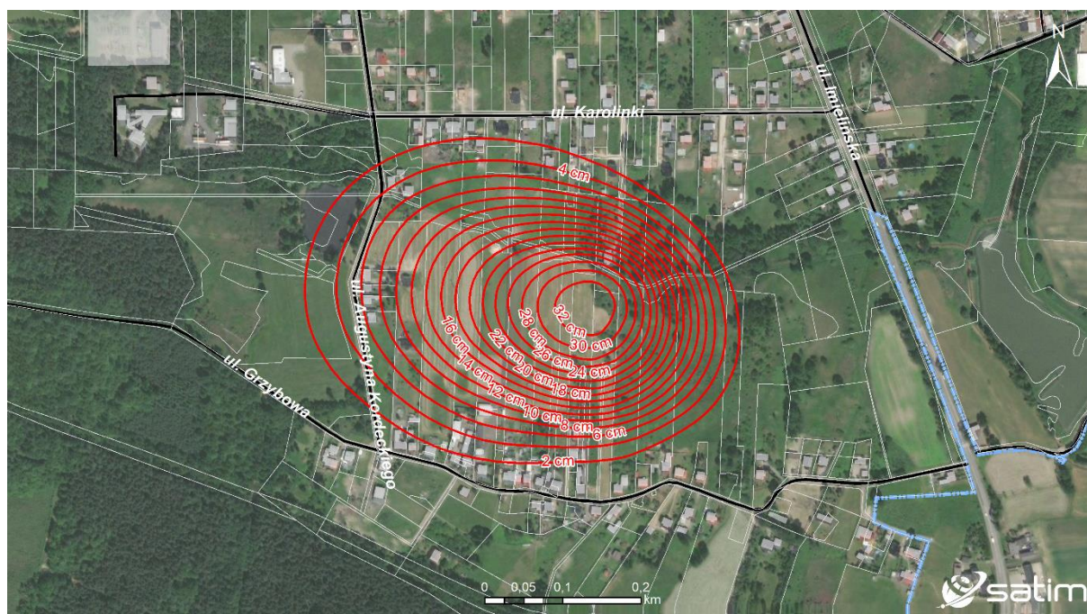
Ryc. 3 - Mapa pionowych przemieszczeń terenu – obniżenia w formie izolinii. Izolinie oddalone od siebie o stałą wartość 2 cm cięcia poziomowego.
