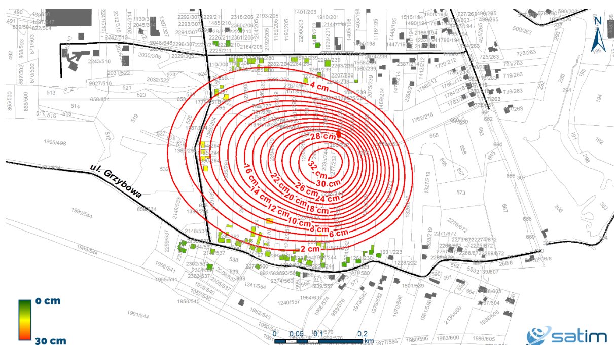
Ryc. 4 - Mapa pionowych przemieszczeń terenu – obniżenia w formie izolinii. Izolinie oddalone od siebie o stałą wartość 2 cm cięcia poziomowego. W II kwartale 2020 r. 53 budynki znajdowały się na zagrożonym obszarze.
