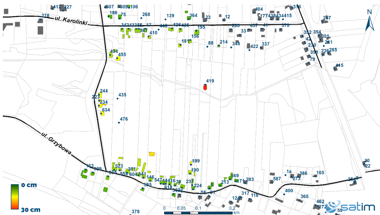
Ryc. 5 - Mapa zagrożonych budynków. Kolorami oznaczone zostały budynki ze względu na wielkość osiadania terenu pod nimi w II kwartale 2020 r.; liczby przy budynkach oznaczają numery adresowe
