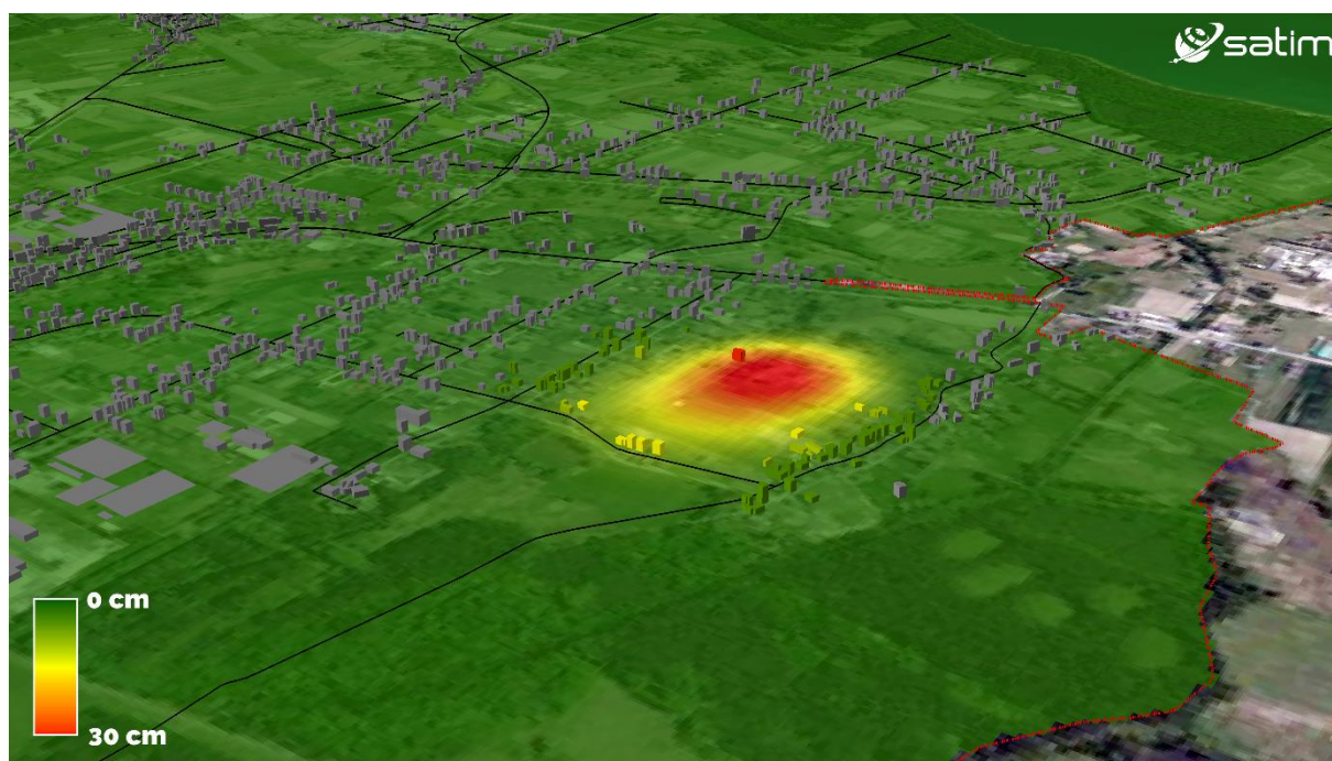
Ryc. 7 – Wizualizacja budynków na niecce obniżeniowej. Kolorami oznaczone zostały budynki ze względu na wielkość osiadania terenu pod nimi w II kwartale 2020 r.
