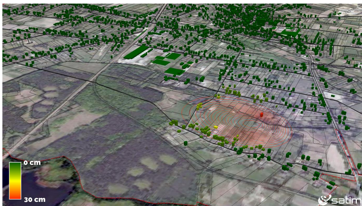
Ryc. 8 – Wizualizacja budynków na niecce obniżeniowej. Kolorami oznaczone zostały budynki ze względu na wielkość osiadania terenu pod nimi w II kwartale 2020 r. Izolinie osiadań oddalone od siebie o stałą wartość 2 cm cięcia poziomowego
