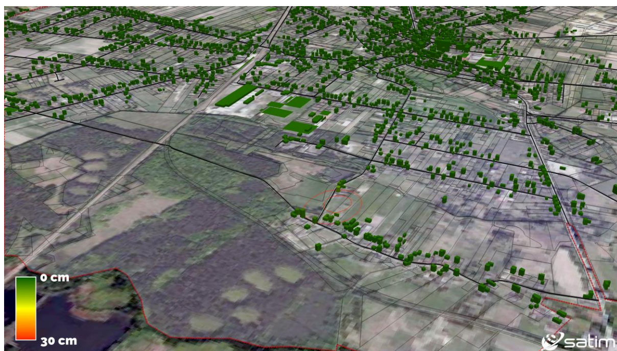
Ryc. 8 – Wizualizacja budynków na niecce obniżeniowej. Kolorami oznaczone zostały budynki ze względu na wielkość osiadania terenu pod nimi w II kwartale 2019r. Izolinie osiadań oddalone od siebie o stałą wartość 1 cm cięcia poziomowego
