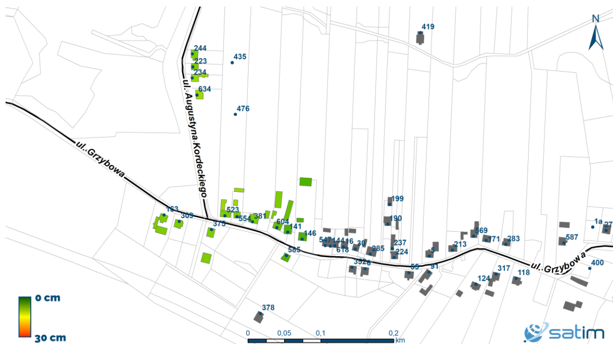
Ryc. 5 - Mapa zagrożonych budynków. Kolorami oznaczone zostały budynki ze względu na wielkość osiadania terenu pod nimi w II kwartale 2019r. Liczby przy budynkach oznaczają numery adresowe.
