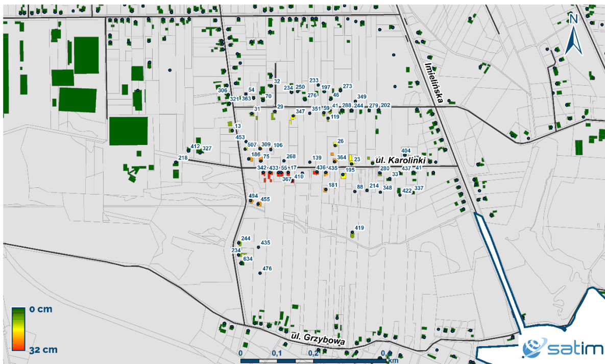
Ryc. 5 - Mapa zagrożonych budynków. Kolorami oznaczone zostały budynki ze względu na wielkość osiadania terenu pod nimi w III kwartale 2021 r.; liczby przy budynkach oznaczają numery adresowe
