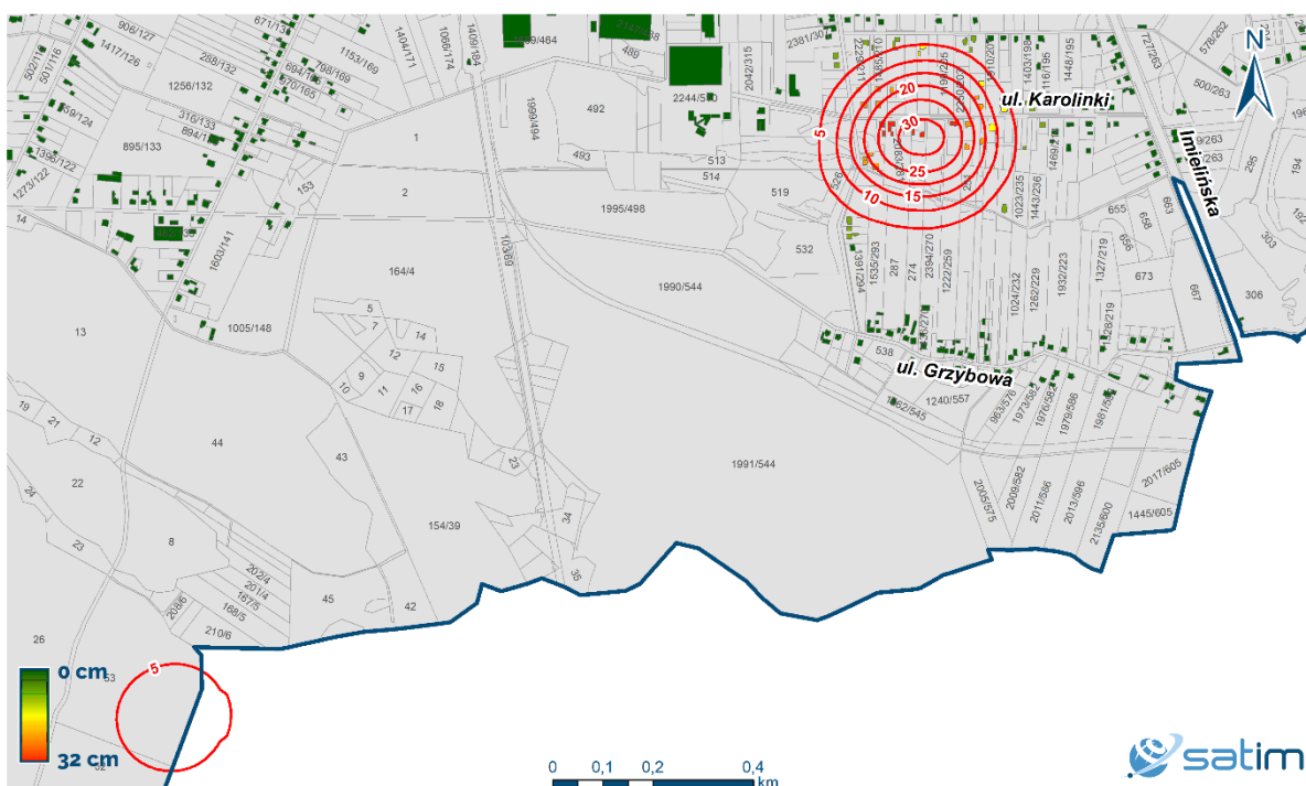
Ryc. 4 - Mapa pionowych przemieszczeń terenu – obniżenia w formie izolinii. Izolinie oddalone od siebie o stałą wartość 5 cm cięcia poziomowego. W III kwartale 2021 r. 58 budynków znajdowało się na zagrożonym obszarze.
