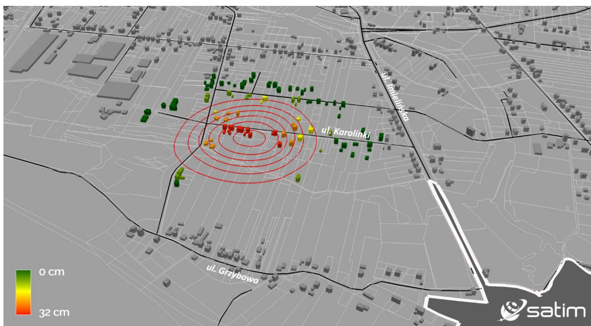
Ryc. 10 – Wizualizacja budynków i ulic. Kolorami oznaczone zostały budynki ze względu na wielkość osiadania terenu pod nimi w III kwartale 2021 r. Izolinie osiadań oddalone od siebie o stałą wartość 5 cm cięcia poziomowego
