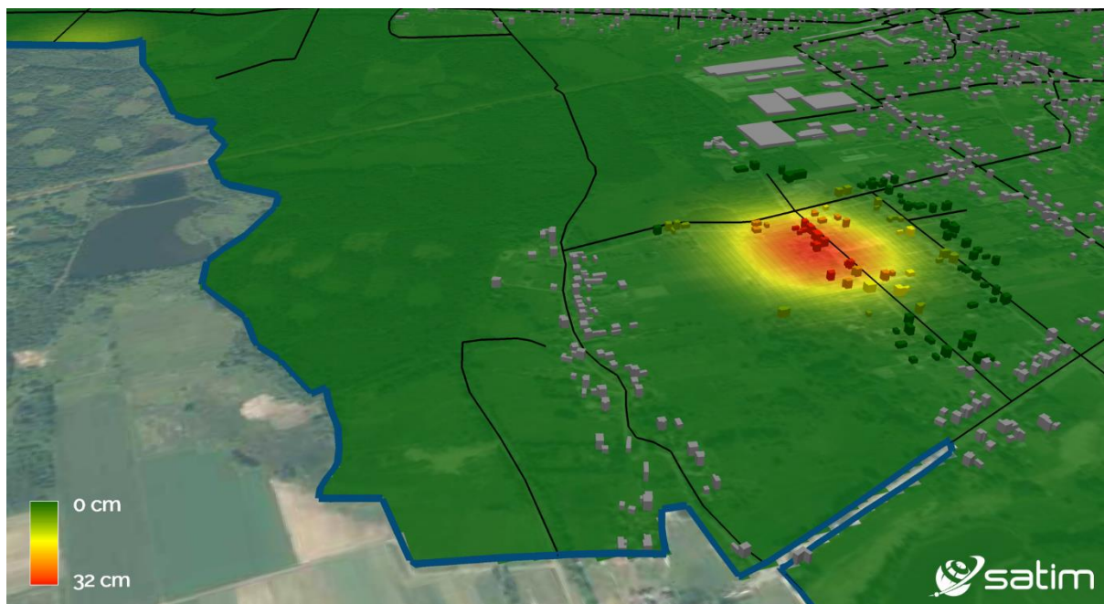
Ryc. 7 – Wizualizacja budynków na niecce obniżeniowej. Kolorami oznaczone zostały budynki ze względu na wielkość osiadania terenu pod nimi w III kwartale 2021 r.
