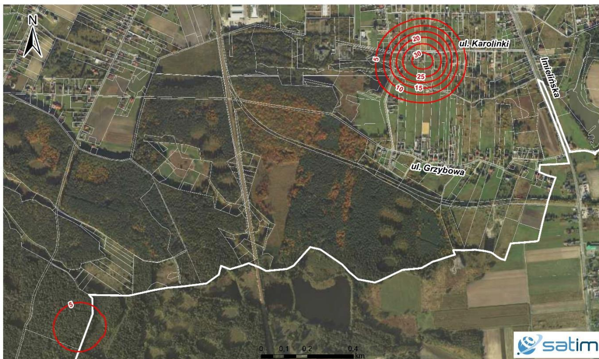
Ryc. 3 - Mapa pionowych przemieszczeń terenu – obniżenia w formie izolinii. Izolinie oddalone od siebie o stałą wartość 5 cm cięcia poziomowego.
