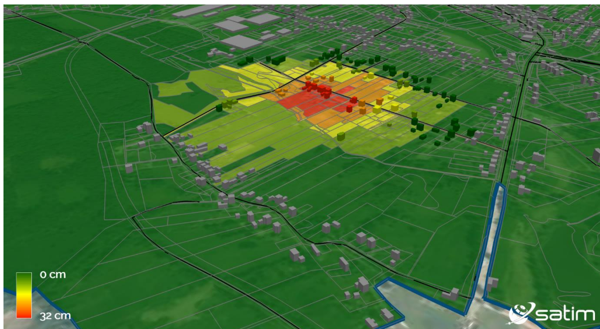
Ryc. 9 – Wizualizacja działek ewidencyjnych objętych osiadaniem terenu. Kolorami oznaczone zostały działki ze względu na średnią wielkość osiadania terenu w ich obrębie.
