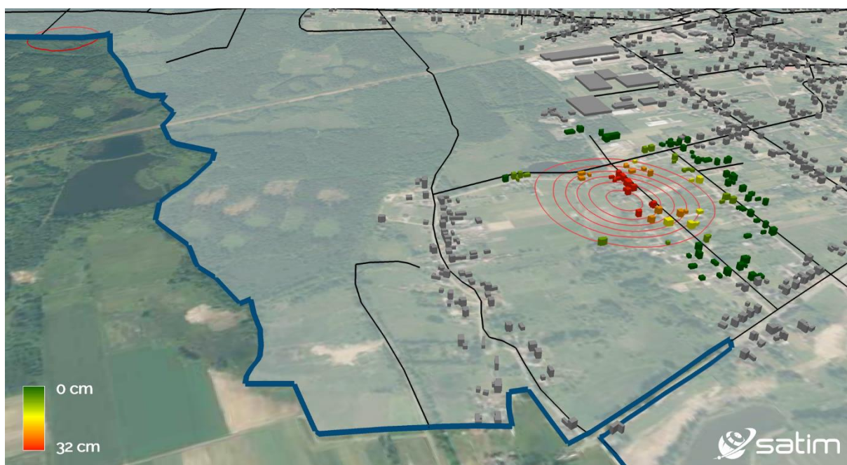
Ryc. 8 – Wizualizacja budynków na niecce obniżeniowej. Kolorami oznaczone zostały budynki ze względu na wielkość osiadania terenu pod nimi w III kwartale 2021 r. Izolinie osiadań oddalone od siebie o stałą wartość 5 cm cięcia poziomowego
