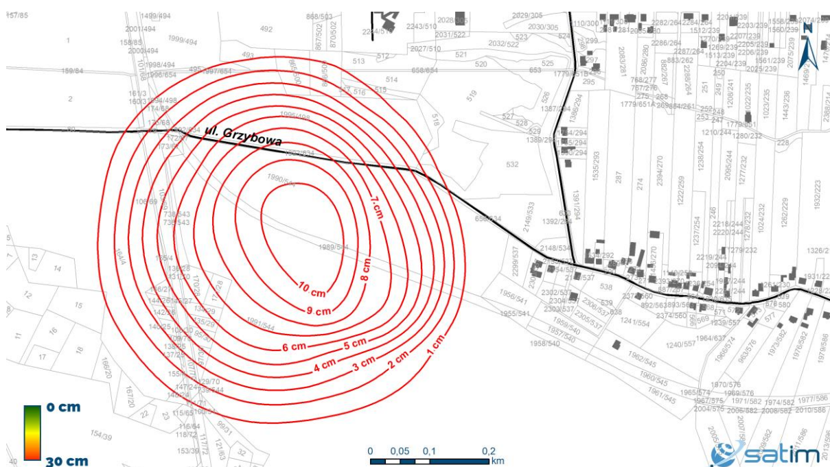
Ryc. 4 - Mapa pionowych przemieszczeń terenu – obniżenia w formie izolinii. Izolinie oddalone od siebie o stałą wartość 1 cm cięcia poziomowego. W III kwartale 2019 r. żaden budynek nie znajdował się na zagrożonym obszarze.
