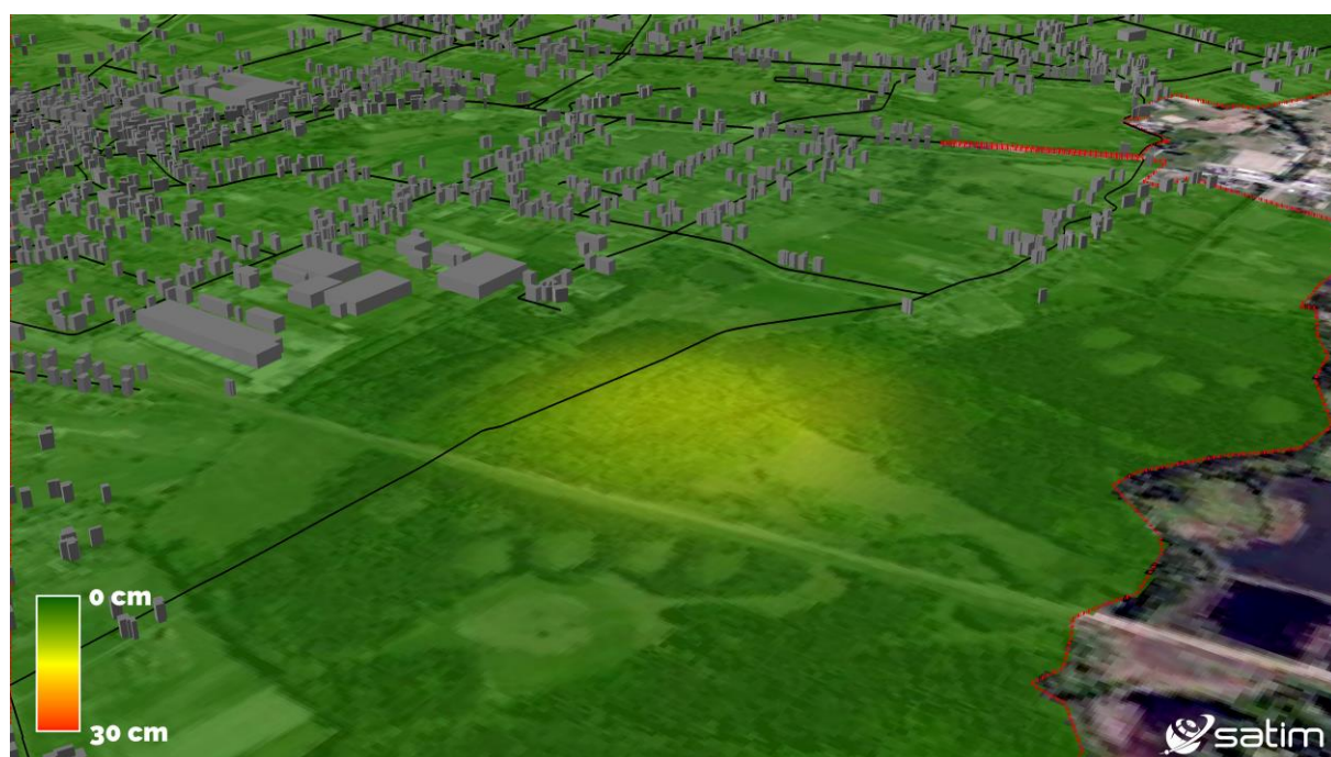
Ryc. 6 - Wizualizacja budynków na niecce obniżeniowej. Kolorami oznaczone zostały budynki ze względu na wielkość osiadania terenu pod nimi w III kwartale 2019r.
