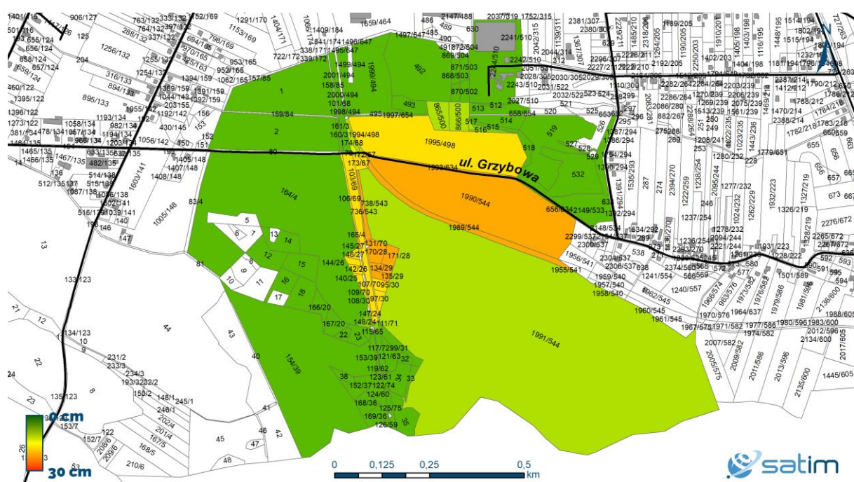
Ryc. 5 - Mapa działek ewidencyjnych. Kolorami oznaczone zostały działki ze względu na średnią wielkość osiadania terenu w ich obrębie.
