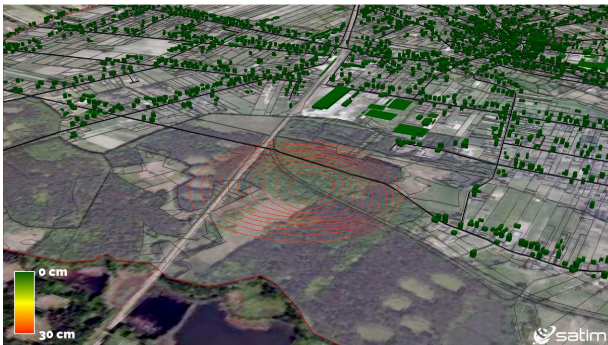
Ryc. 7 – Wizualizacja budynków na niecce obniżeniowej. Kolorami oznaczone zostały budynki ze względu na wielkość osiadania terenu pod nimi w III kwartale 2019 r. Izolinie osiadań oddalone od siebie o stałą wartość 1 cm cięcia poziomowego
