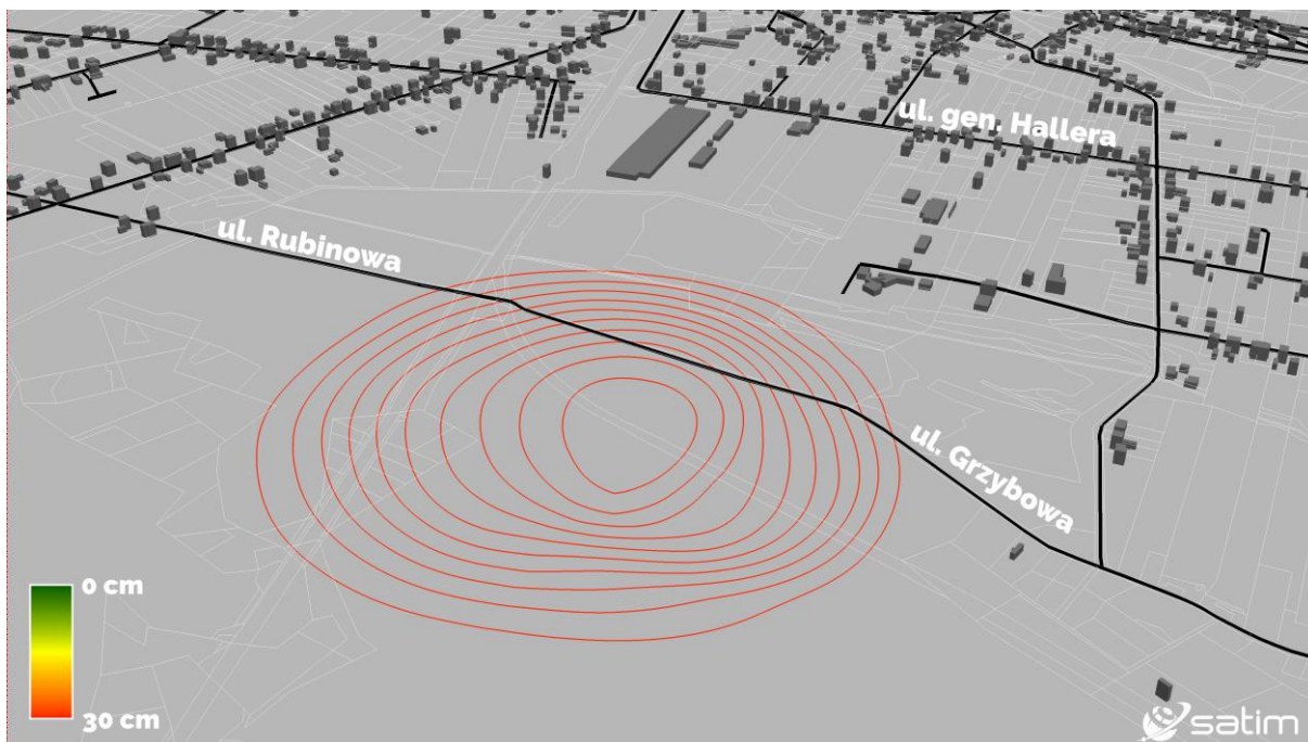
Ryc. 9 – Wizualizacja budynków i ulic. Kolorami oznaczone zostały budynki ze względu na wielkość osiadania terenu pod nimi w III kwartale 2019r. Izolinie osiadań oddalone od siebie o stałą wartość 1 cm cięcia poziomowego
