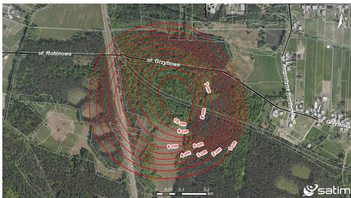
Ryc. 3 - Mapa pionowych przemieszczeń terenu – obniżenia w formie izolinii. Izolinie oddalone od siebie o stałą wartość 1 cm cięcia poziomowego.
